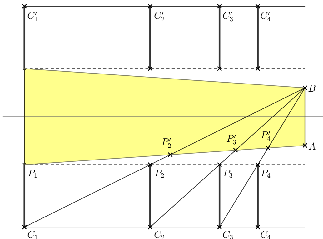
Obrázek 8: Náčrt k určení polohy clon pro zvolené rozměry vyráběného dalekohledu.
