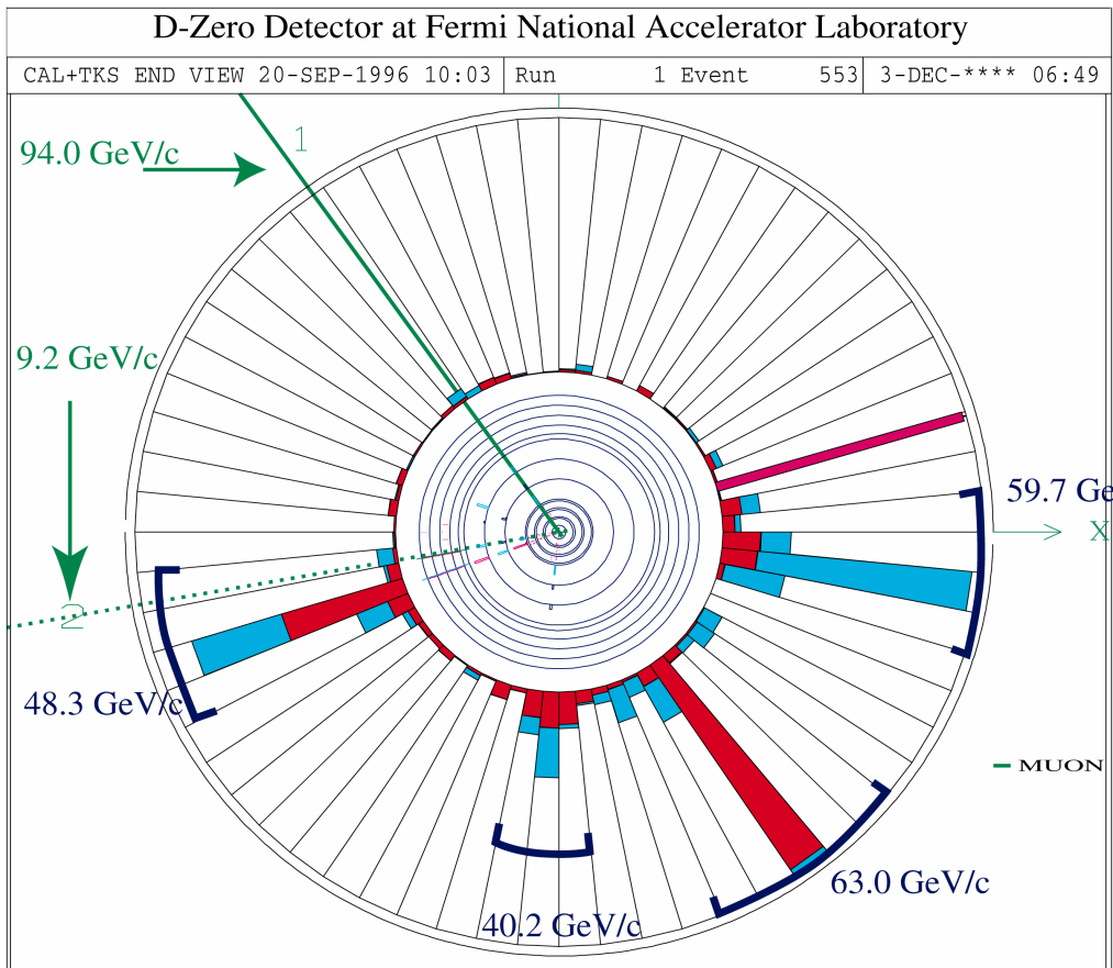
Obr. A.7: Kolmý průřez detektorem (CAL+TKS END VIEW), zobrazena událost 553
