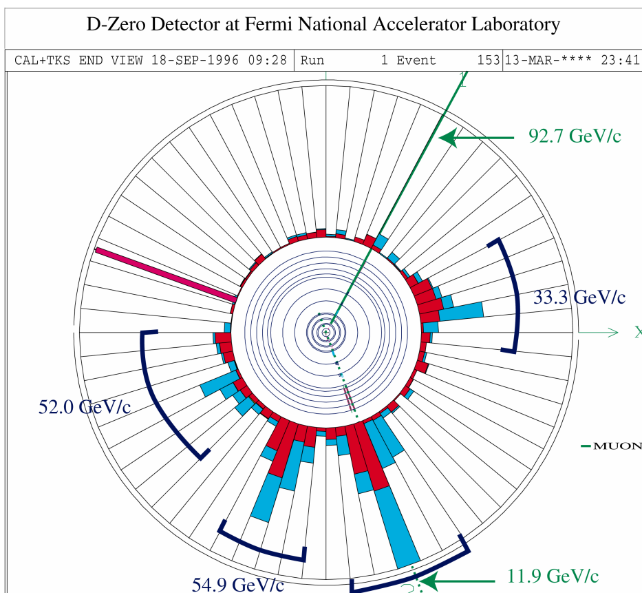
Obr. A.6: Kolmý průřez detektorem (CAL+TKS END VIEW), zobrazena událost 153
