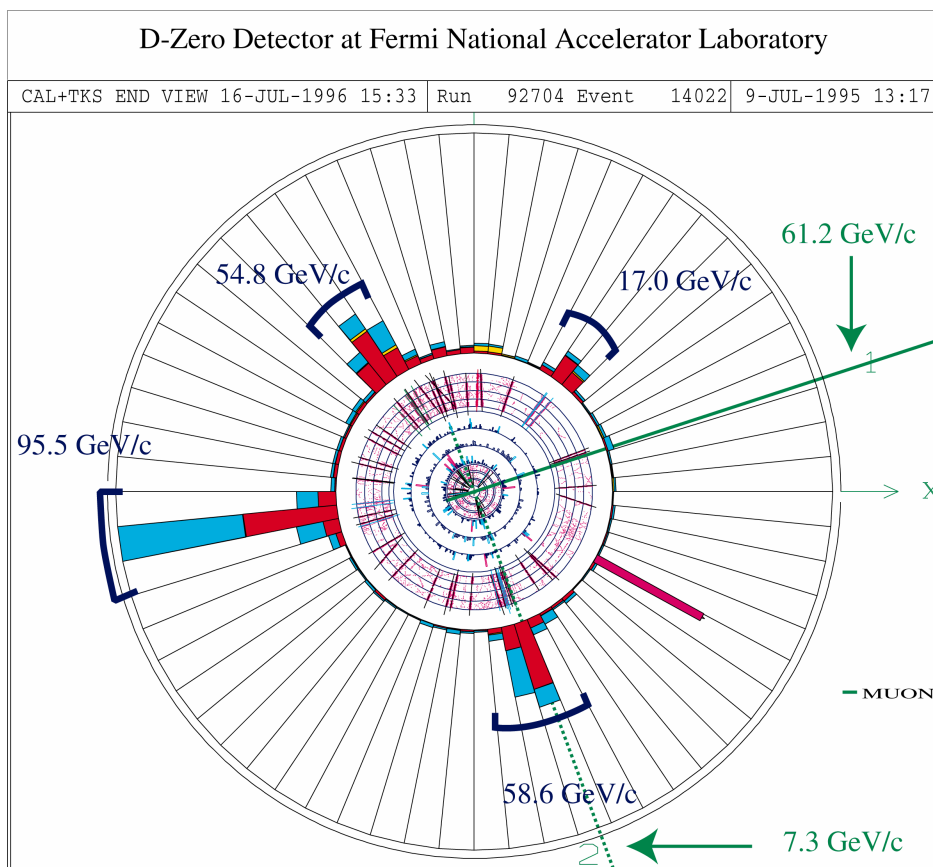
Obr. A.5: Kolmý průřez detektorem (CAL+TKS END VIEW), zobrazena událost 14022
